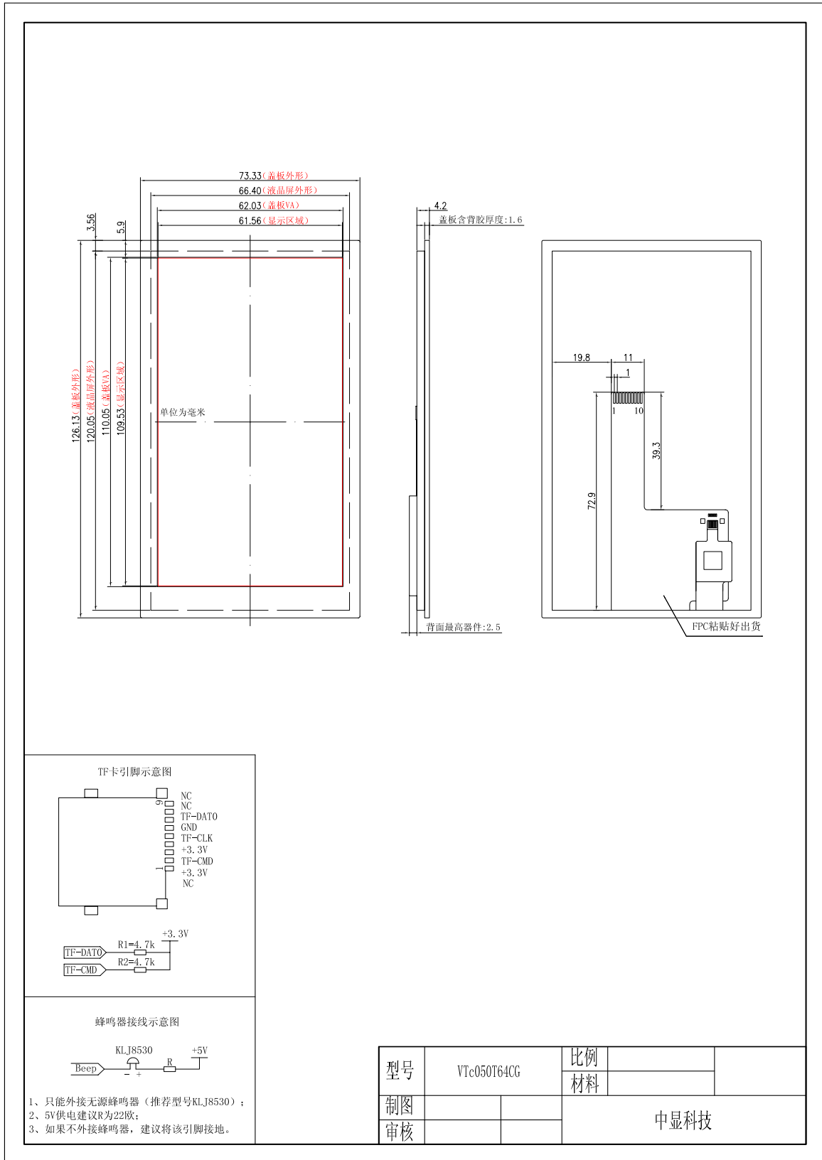
图 3 VTc050T64CG 尺寸图
