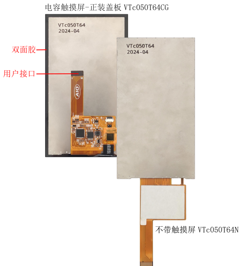
图 1 产品外观及硬件配置图
