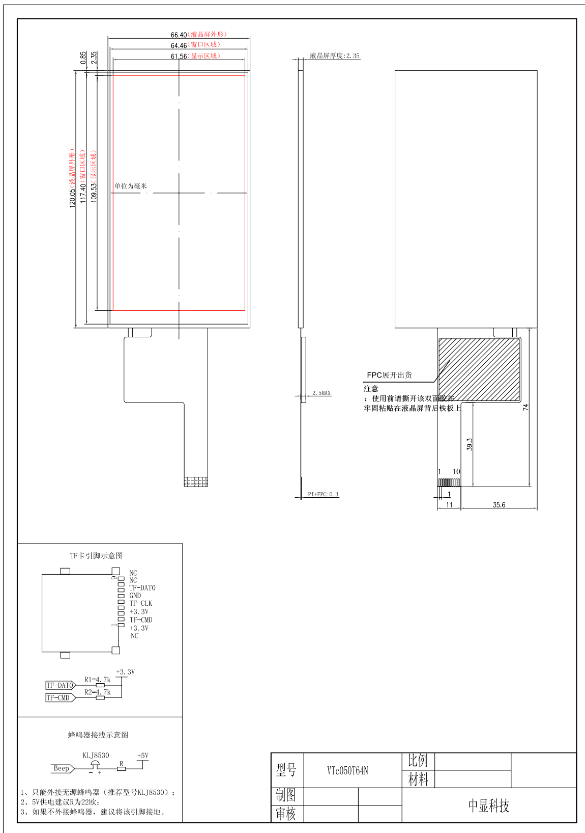
图 2 VTc050T64N 尺寸图
